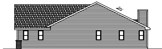
Right Elevation
